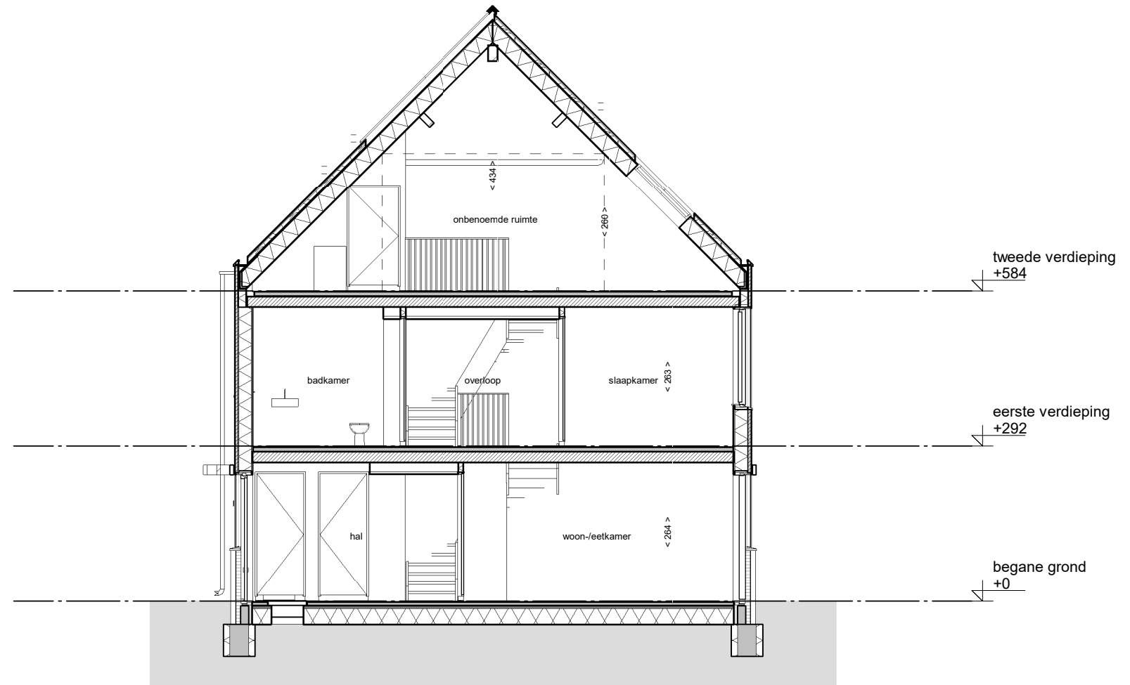
doorsnede
